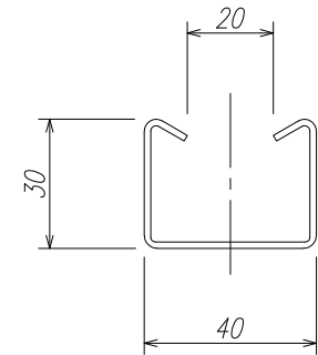
レール詳細図 S=1/2
