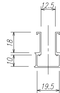
レール詳細図 S=1/2
