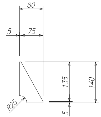
補強リブ詳細図
