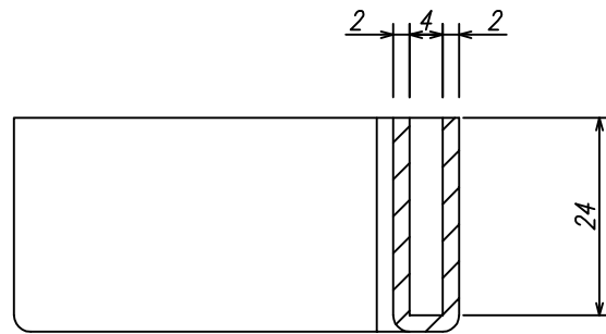
A-A 断面図
