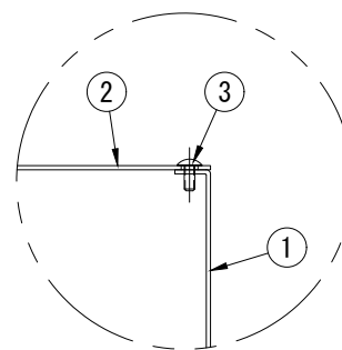
ふた取付部詳細図
